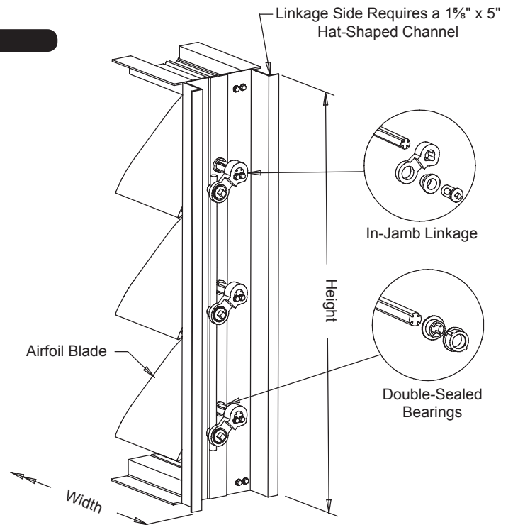
A28 (Parallel Blade)
